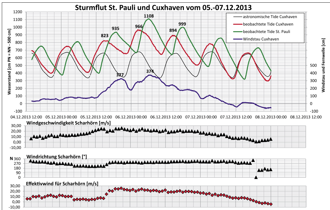
Abb. 5: Sturmflut- und Windverlauf vom 4. bis 8. Dezember 2013
