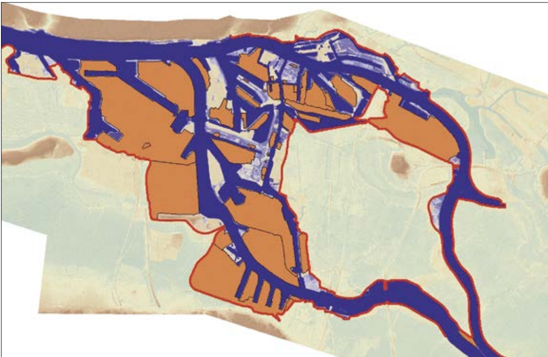
Abb. 16: Durch private Hochwasserschutzanlagen geschützte Flächen und Überflutungssituation bei NN + 6,08 m im Hamburger Hafen
